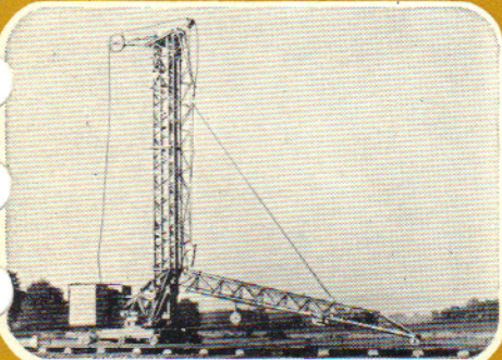
Grue pré-cablée : pas de mât rallonge
