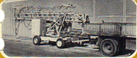
Transport : 4 roues, timon d'attelage
