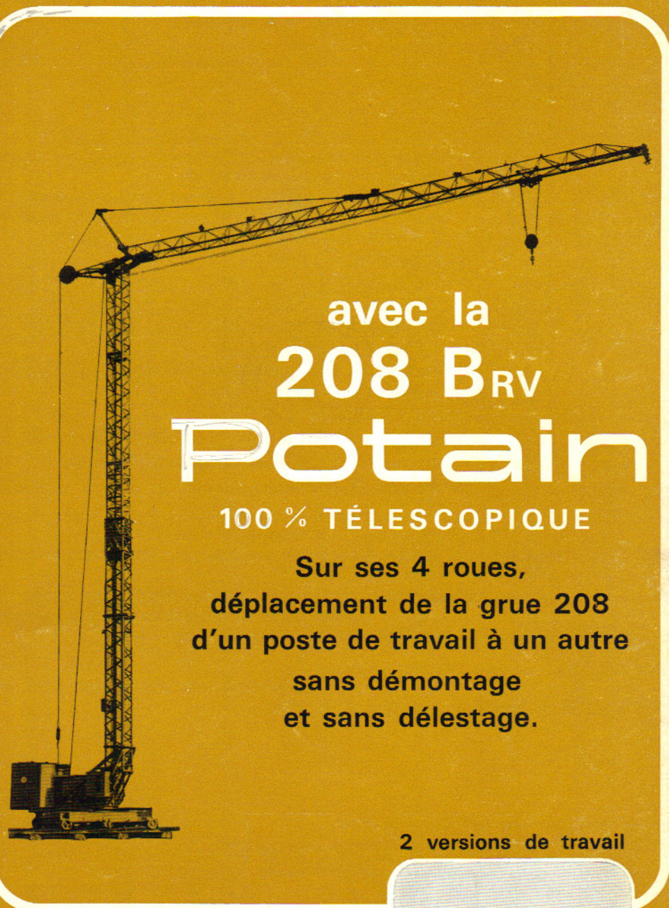
Dépliage de flèche dans 2 plans (Breveté)
