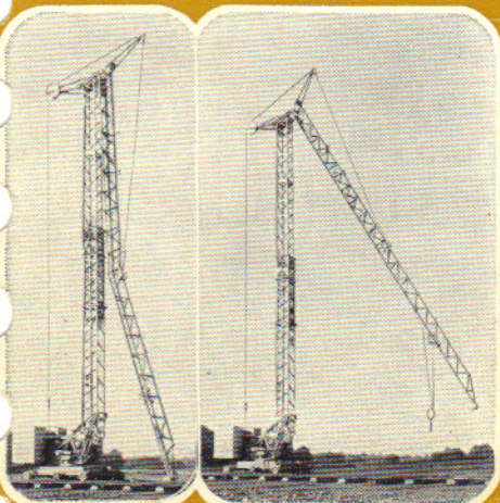
Verrouillage automatique de la mâture
