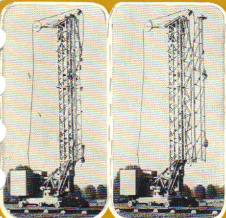
Dépliage de flèche dans 2 plans (Breveté)
